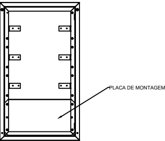
VISTA FRONTAL INTERNA NWP-418-S COM SESSÃO DE PLACA
