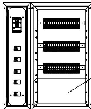
VISTA FRONTAL INTERNA WH-4-DG-S+NWP-418-S CONJUNTO ACOPLADO DISJUNTORES , GERAL CAIXA MOLDADA, BLOCO DE DISTRIBUIÇÃO E SESSÃO DE PLACA
