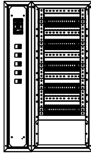
VISTA FRONTAL INTERNA NWP-6-DG-S + NWP-618-S COM MINIDISJUNTORES E SESSÃO DE PLACA
