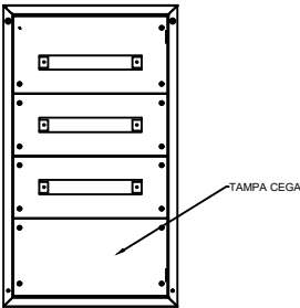
VISTA FRONTAL INTERNA NWP-418-S COM TAMPA CEGA
