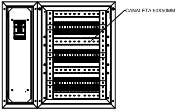
VISTA FRONTAL INTERNA NWP-318-S +NWP-3-DG-S CONJUNTO ACOPLADO, DISJUNTORES E GERAL CAIXA MOLDADA
