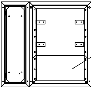
VISTA FRONTAL INTERNA NWP-3-DG-S+NWP-318-S COM SESSÃO DE PLACA
