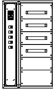
VISTA FRONTAL INTERNA NWP-6-DG-S + NWP-618-S COM TAMPAS ABERTAS E TAMPA CEGA
