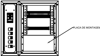
VISTA FRONTAL INTERNA NWP-3-DG-S+NWP-318-S CONJUNTO ACOPLADO DISJUNTORES, BORNES E SESSÃO DE PLACA
