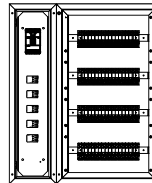
VISTA FRONTAL INTERNA NWP-4-DG-S+NWP-418-S CONJUNTO ACOPLADO DISJUNTORES , GERAL CAIXA MOLDADA, BORNES E BLOCO DE DISTRIBUIÇÃO
