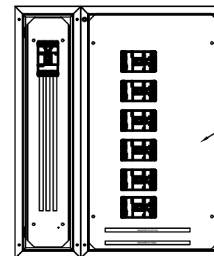
VISTA FRONTAL INTERNA NWP-4-DG-S+NWP-418-S-PM CONJUNTO ACOPLADO GERAL CAIXA MOLDADA E DISJUNTORES DISTRIBUIÇÃO CAIXA MOLDADA
