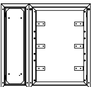
VISTA FRONTAL INTERNA CONJUNTO ACOPLADO NWP-318-S + NWP-3-DG-S
