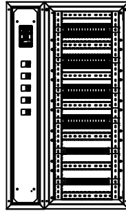
VISTA FRONTAL INTERNA NWP-6-DG-S + NWP-618-S COM MINIDISJUNTORES E BORNES
