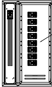
VISTA FRONTAL INTERNA NWP-6-DG-S + NWP-618-S-PM GERAL CAIXA MOLDADA E DISJUNTORES DE DISTRIBUIÇÃO CAIXA MOLDADA
