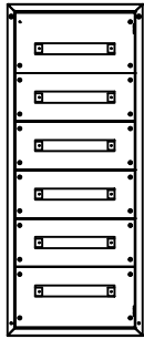
VISTA FRONTAL INTERNA NWP-618-S TAMPAS ABERTAS
