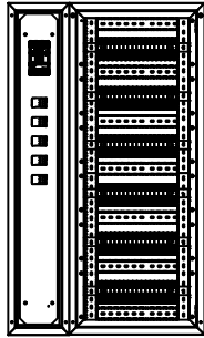
VISTA FRONTAL INTERNA NWP-6-DG-S + NWP-618-S COM MINIDISJUNTORES
