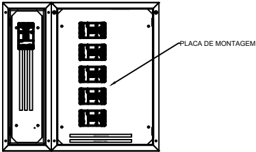
VISTA FRONTAL INTERNA NWP-3-DG-S+NWP-318-S-PM CONJUNTO ACOPLADO DISJUNTORES CAIXA MOLDADA
