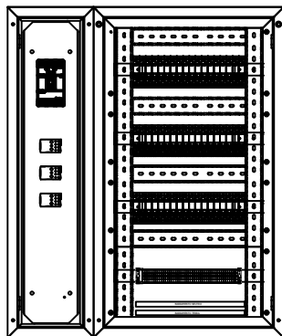
VISTA FRONTAL INTERNA NWP-4-DG-S+NWP-418-S CONJUNTO ACOPLADO DISJUNTORES , GERAL CAIXA MOLDADA, BORNES E BLOCO DE DISTRIBUIÇÃO
